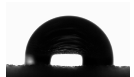
Abb. 1: Wasserkontaktwinkel einer Folienprobe mit HMDSO-Beschichtung, die eine erhöhte Hydrophobizität der Oberfläche zeigt (WCA > 90°)
