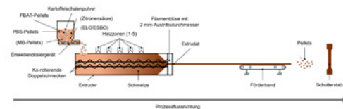
Abb. 1: Versuchsaufbau bei der Herstellung von Schulterstäben aus PBS-/PBAT-Blends mit verschiedenen Kartoffelschalenanteilen und unterschiedlichen Additiven
