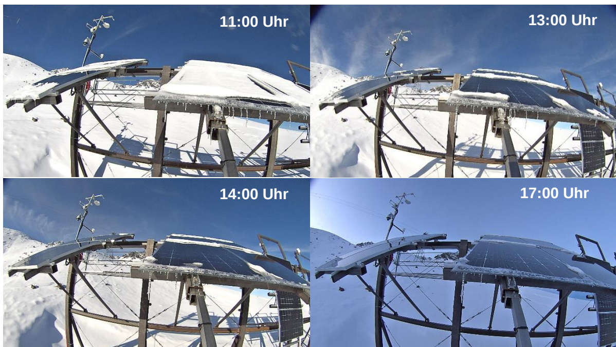
Abbildung 29: Tagesbeispiel für die Schneebedeckung der Segmente A und B zum Vergleich mit Abbildung 28 (01. Dezember 2018). Segment A links, Segment B rechts.
