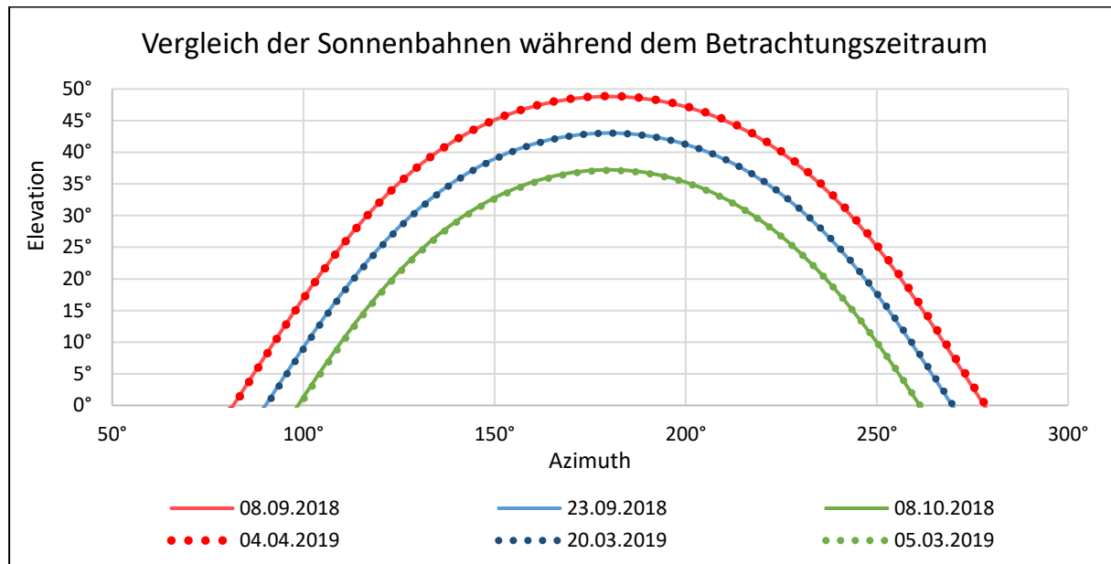
Abbildung 2: Vergleich der Sonnenbahnen während der Tagundnachtgleiche am 20. März und 23. September sowie 15 Tage davor und danach am Standort Davos.
