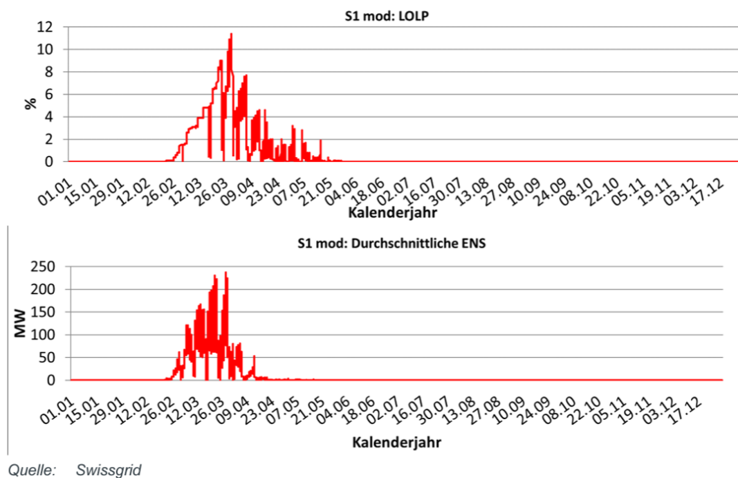
Abbildung 9 LOLP und ENS im Szenario «Keine Kooperation»
