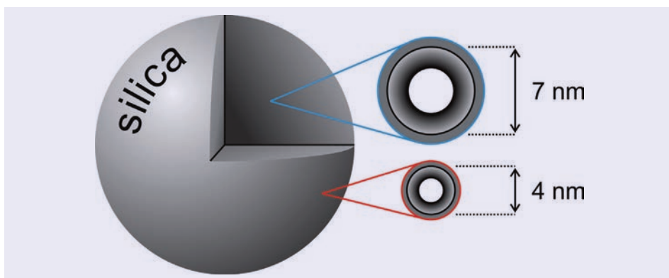
Abb. 2: Schematische Darstellung von kugelförmigen Silica-Partikeln mit Engpässen an den Nanokanaleingängen. 4
