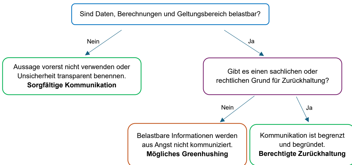
Abbildung 3: Entscheidungsbaum Greenhushing
