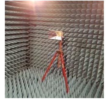
Antennenmesskammer
