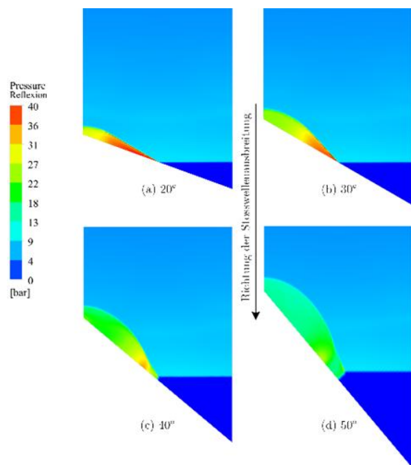
Studie zur Reflexion von Stosswellen bei schiefwinkligem Auftreffen auf Wänden.
