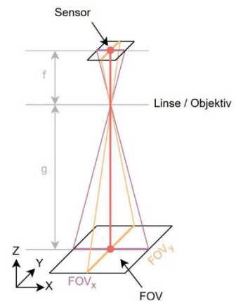
Schematische Darstellung des Aufbaus des Teilsystems Kamera
