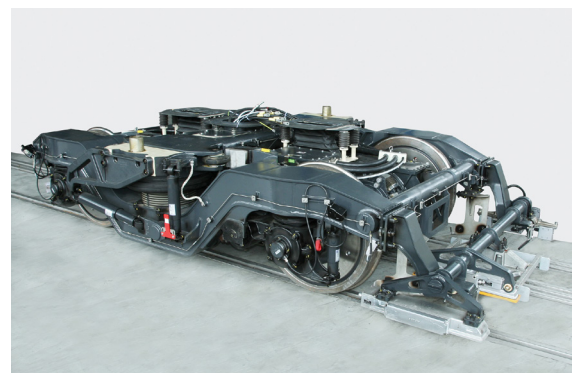
Drehgestell Dosto
